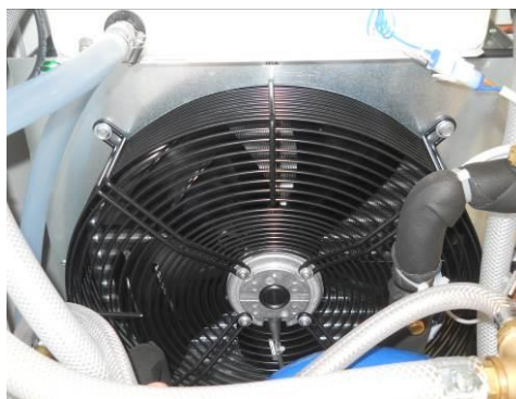
Рис. 19 – Положение вентилятора
