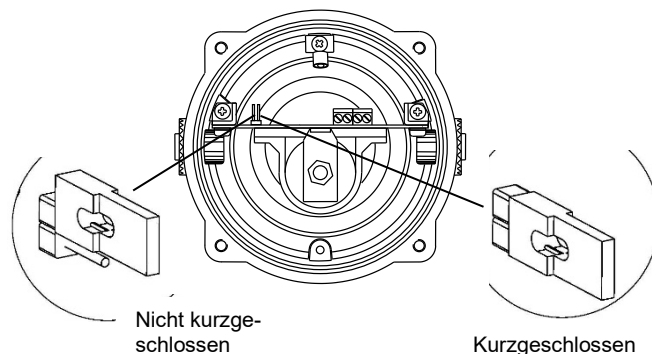
Abb. 6 Steckbrückenkonfiguration
