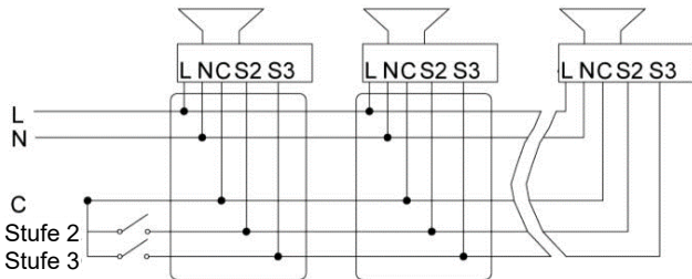
Abb. 3 BExS110 AC Vereinfachtes Blockdiagramm
