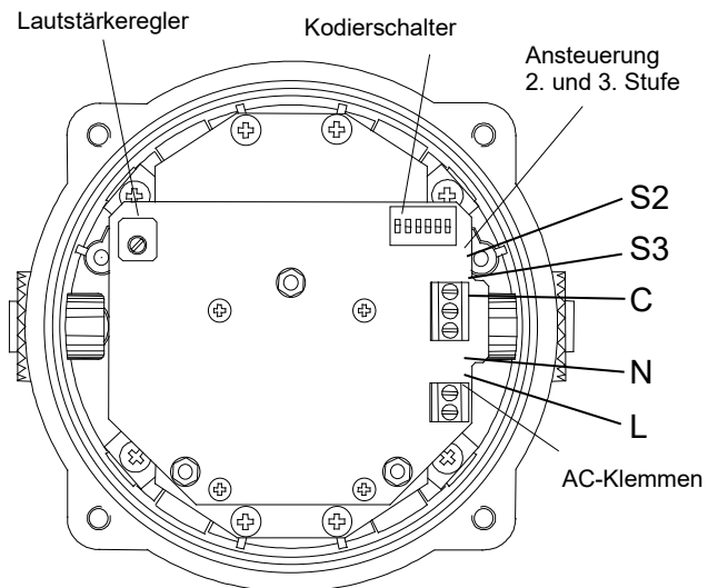
Abb. 4 Klemmen AC-Version
