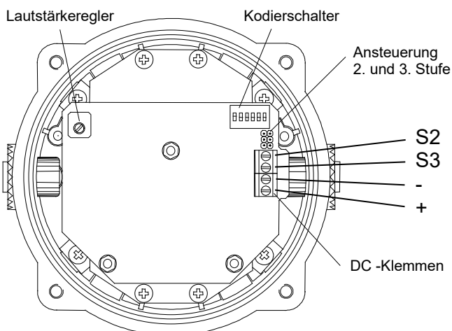
Abb. 6 DC-Version
