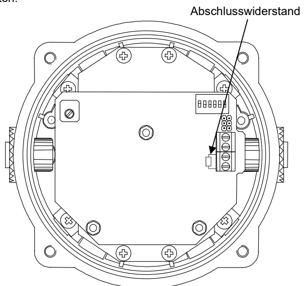
Abb. 8 Position des Abschlusswiderstandes
