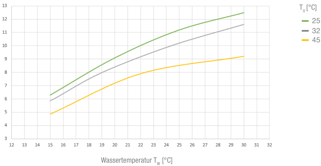
Kälteleistung VLV 12 Q_0 [kW]
