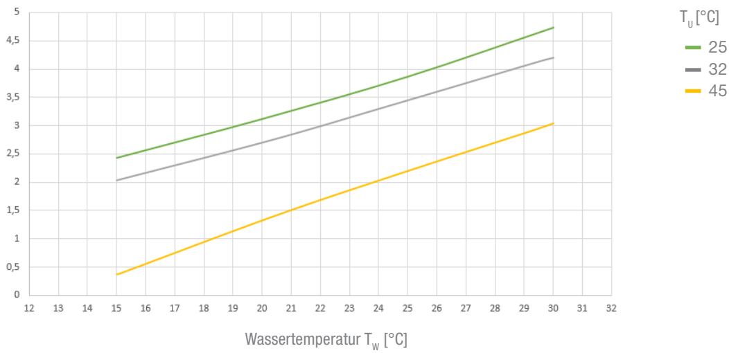
Kälteleistung VLV 4 Q_0 [kW]
